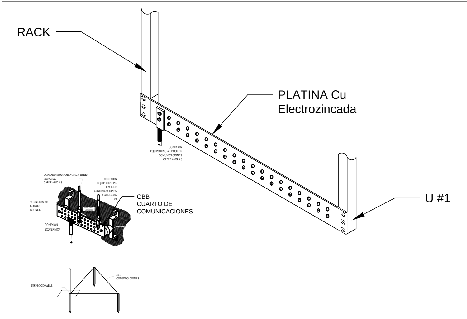
CONEXION A TIERRA RACK
