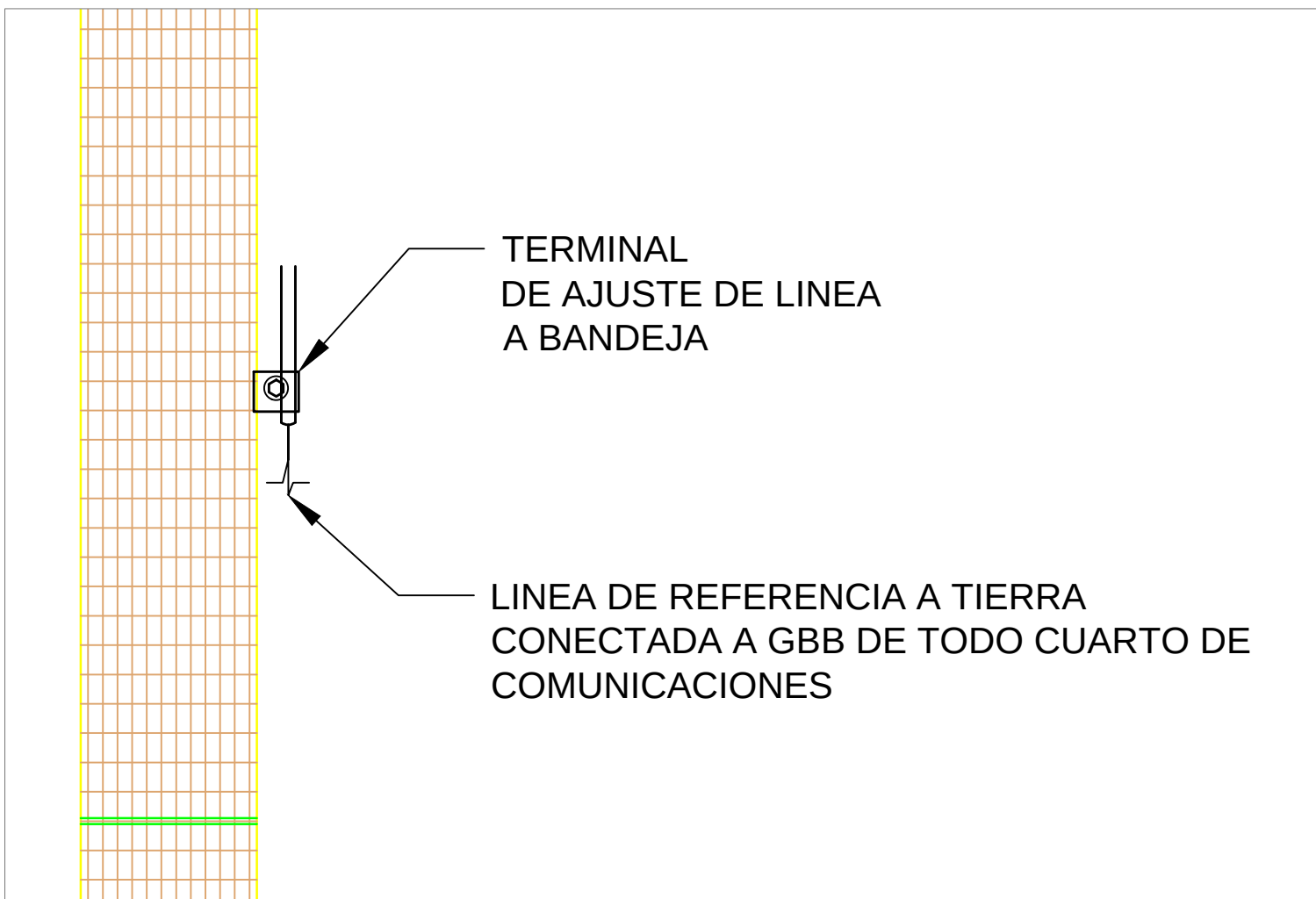
CONEXION A TIERRA BANDEJA
